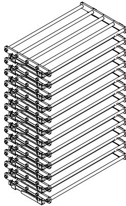
KIT 12 CASSETTI CON BOTTIGLIE LATO LUNGO KIT 12 DRAWERS BOTTLES LONG SIDE
